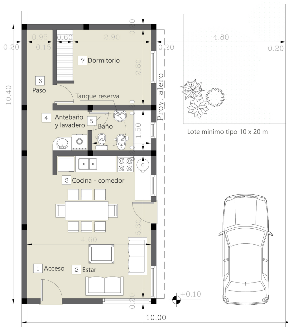
OPCION 1 DORMITORIO Superficie construible: 52.00m 2
