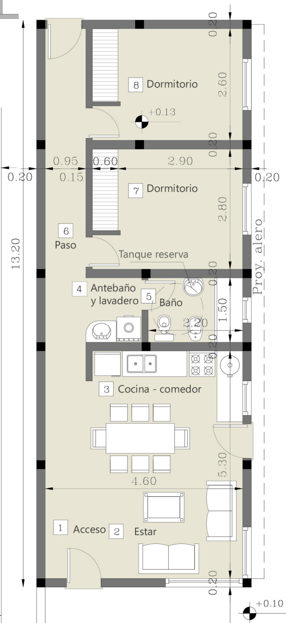
OPCION 2 DORMITORIOS Superficie construible: 66.00m 2
